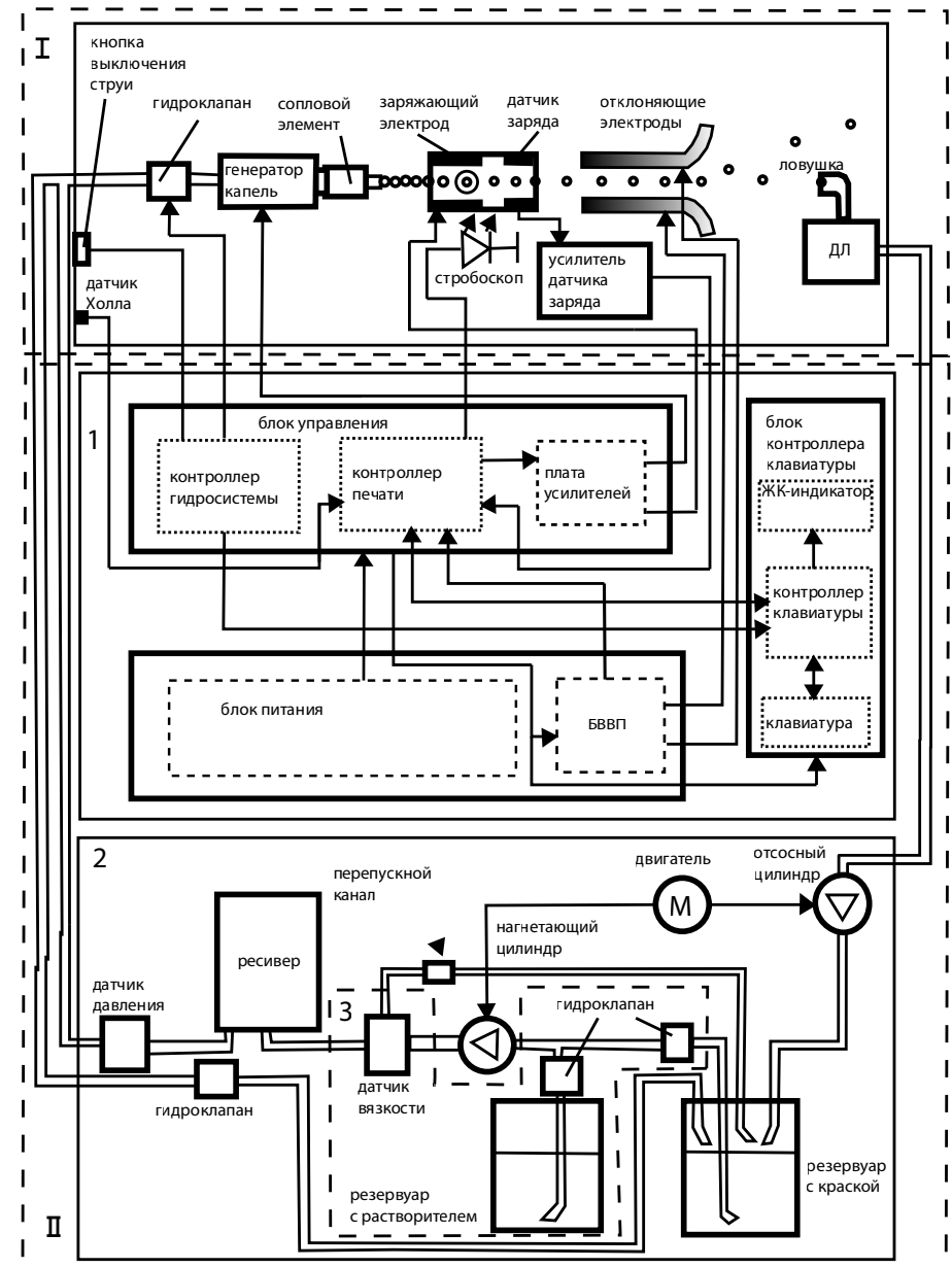
Рис. 2. Функциональная схема маркиратора
